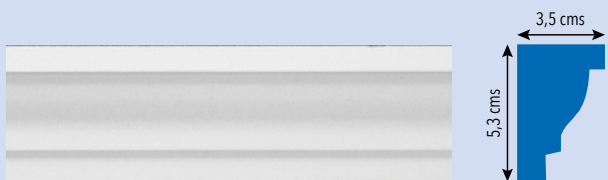
LONGITUD: 101 cms REF: 1054 MOD: P. PALOMA MINI
