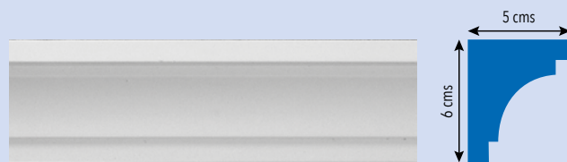
LONGITUD: 100 cms REF: 1049 MOD: MEDIA CAÑA MEDIANA 1
